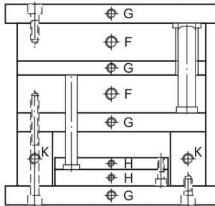
大水口系統 Side Gate System
